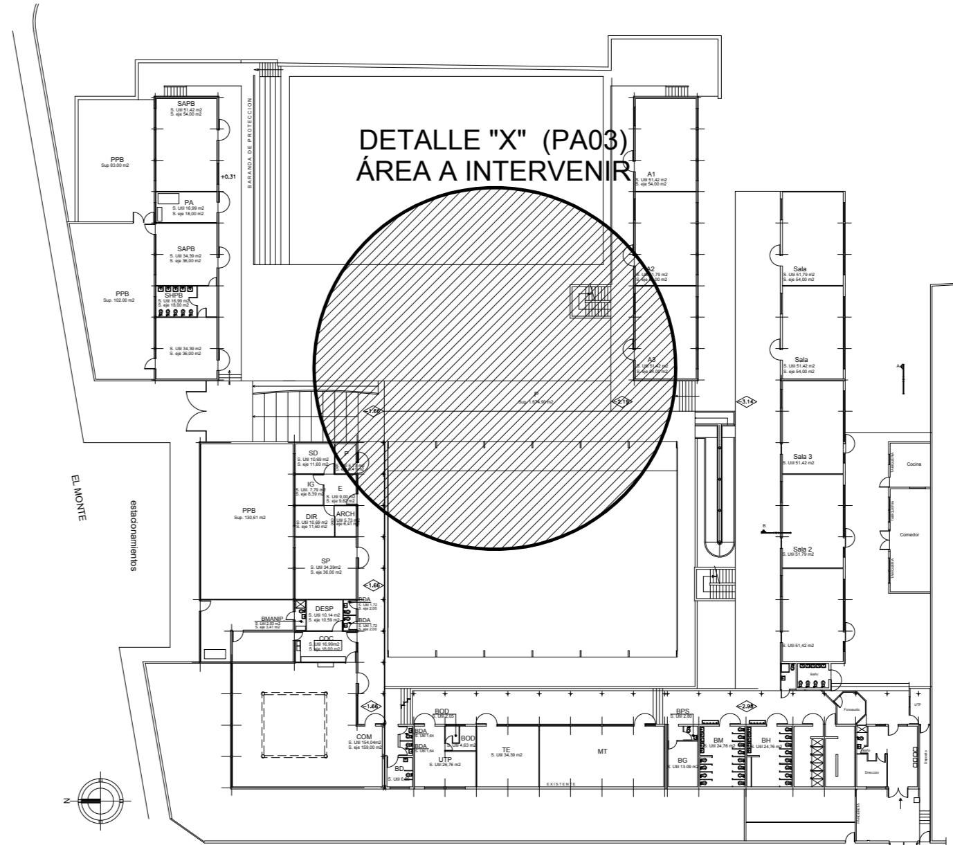
UBICACIÓN ESCALA 1: 500
