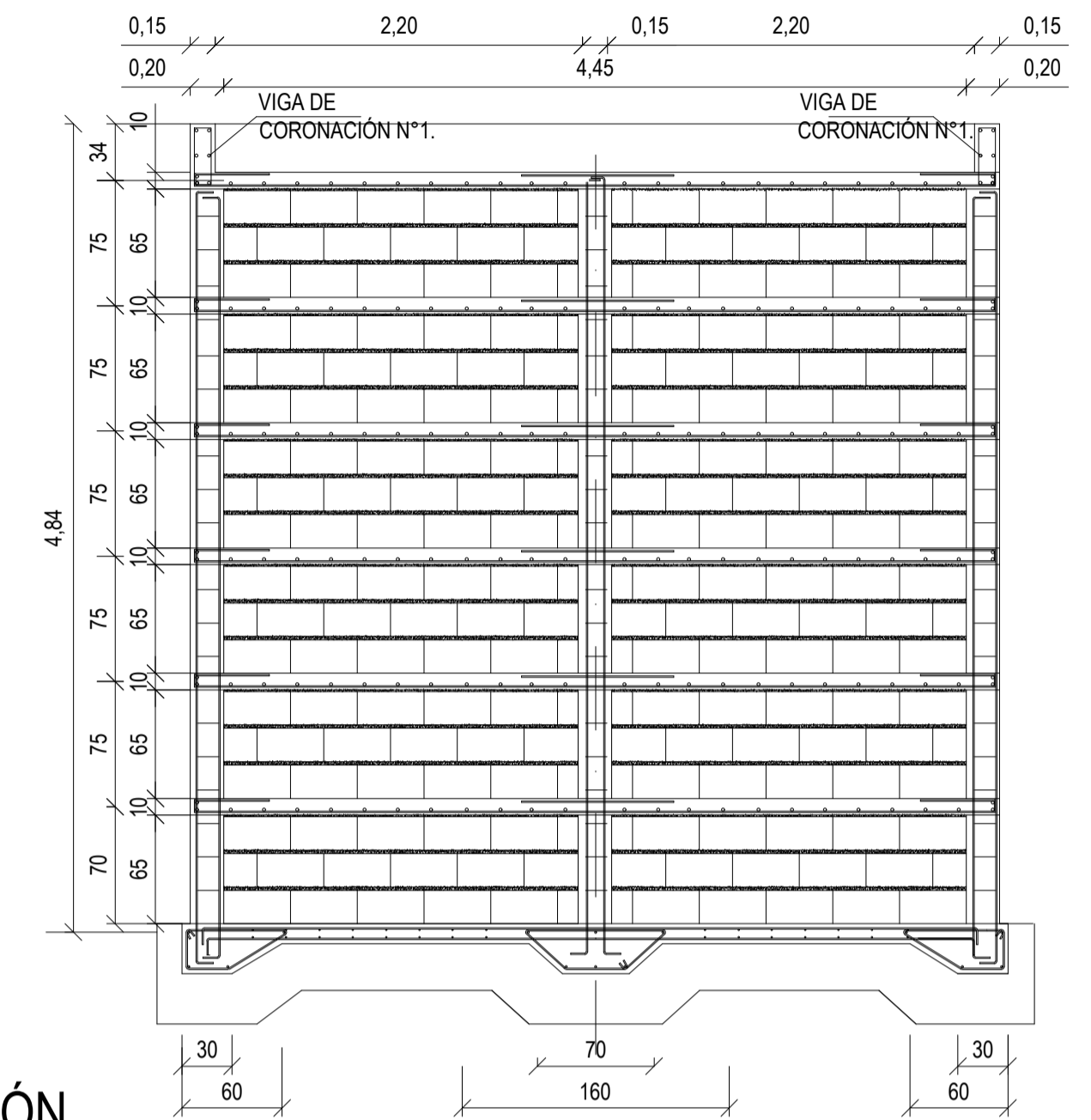
ELEVACIÓN ESCALA 1/50
