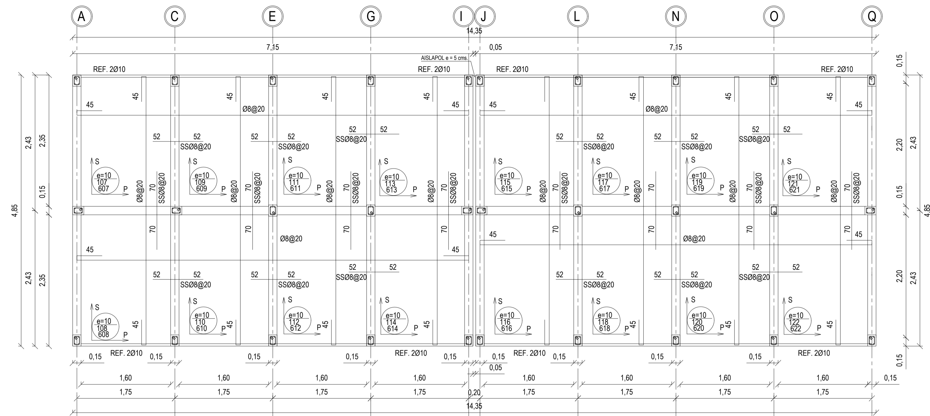
PLANTA DE LOSA TIPO ESCALA 1/50
