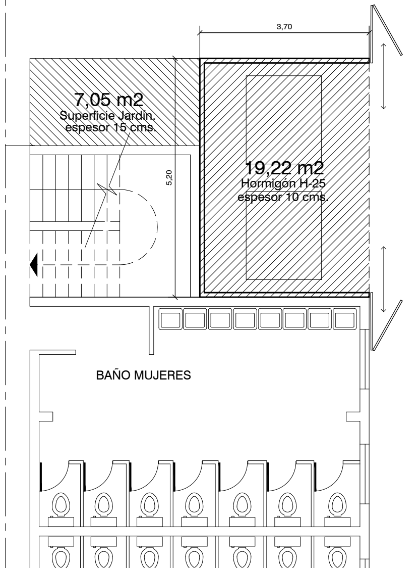
DETALLE "X" EMPLAZAMIENTO DE CASETA DE BASURA. ESCALA 1 : 5 0
