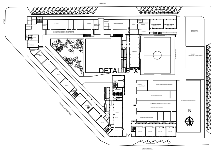
PLANTA BASE 1º PISO ESCALA 1 : 1 0 0 0
