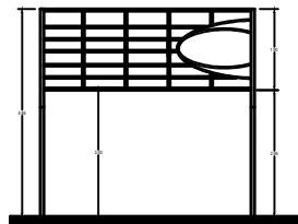
CORTE TRANSVERSAL B-B" ESC. 1:50
