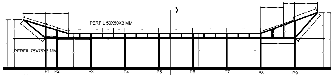
CORTE LONGITUDINAL SOMBREADERO A-A" ESC. 1:50
