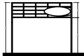
VISTA FRONTAL ACCESO ESC. 1:50
