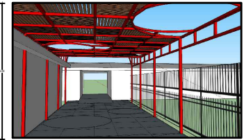
VISTA 3D INTERIOR PASILLOTECHADO
