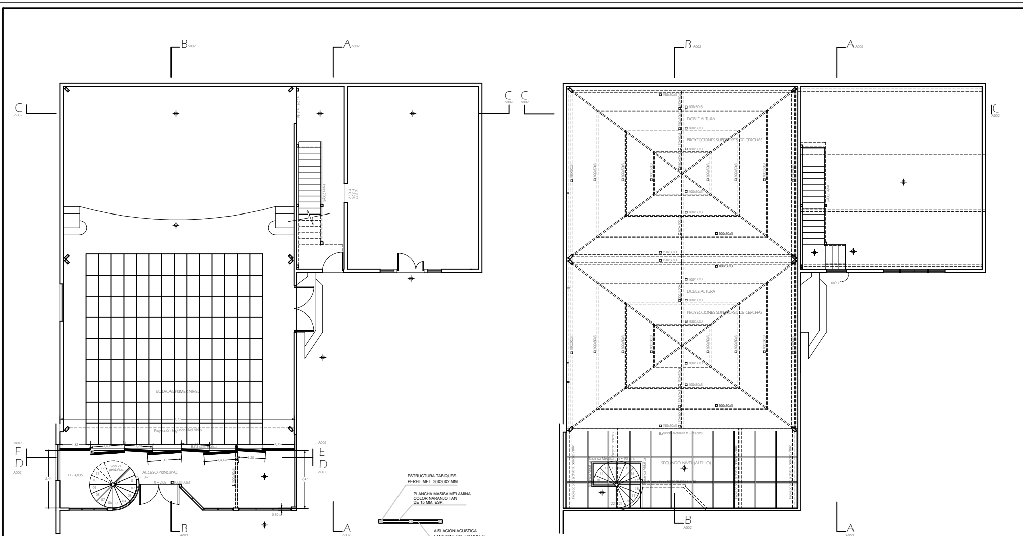
PLANTA PROYECTADA SEGUNDO NIVEL. ESCALA 1 : 50 CON PROYECCION DE NUEVAS CERCHAS DE METALCOM A INSTALAR
