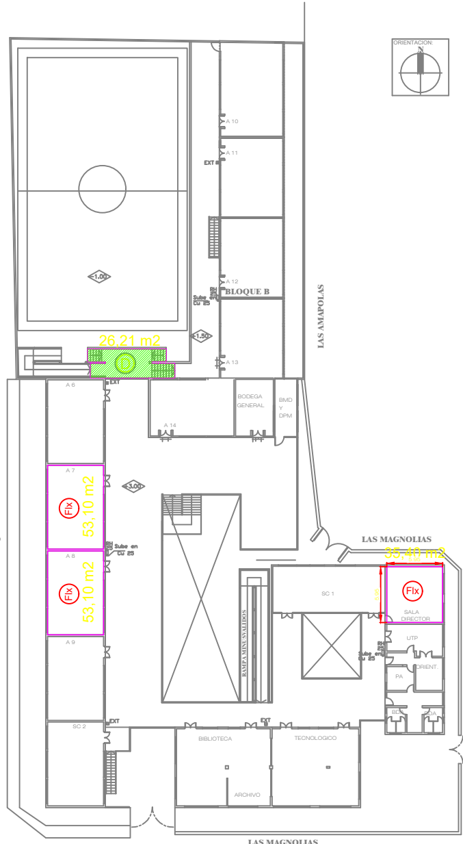
PLANTA. SEGUNDO PISO ESC. 1:200
