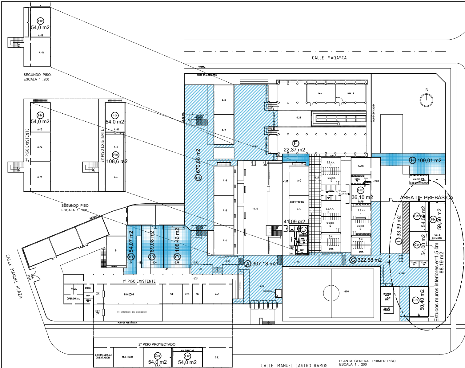
PLANTA GENERAL PRIMER PISO. ESCALA 1 : 200
