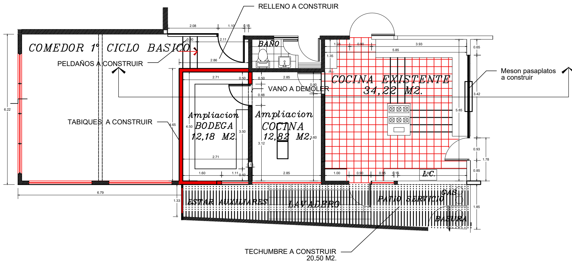
PLANTA GENERAL 1º NIVEL CON INTERVENCIONES MARZO 2017 - AMPLIACION COMEDORES-COCINA Y BODEGA PATRICIO LYNCH D-90
